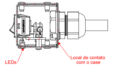
SEÇÃO A-A ESCALA 1 : 2
